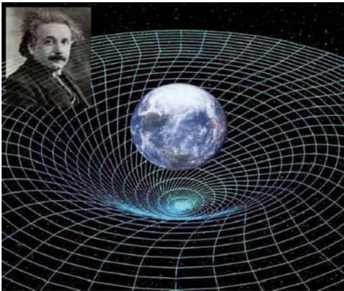
L'Espace-temps d'Einstein
