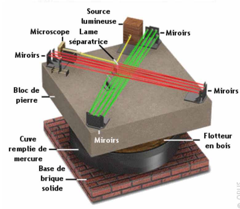
Illustration IV L'interféromètre de Michelson et Morley
